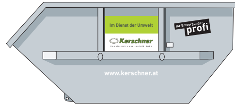
Normmulde 10 m 3 L 410 x B 190 x H 180 cm
